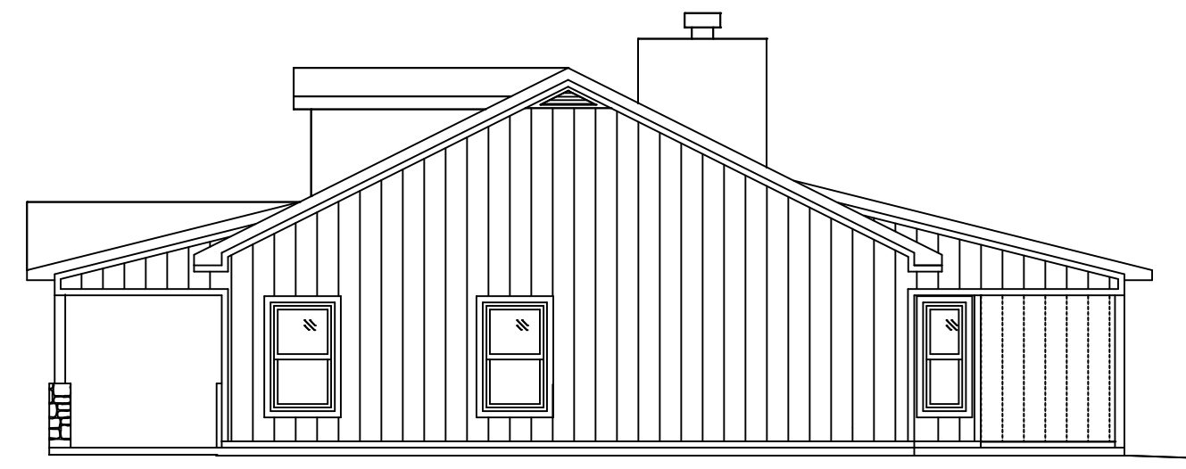
RIGHT ELEVATION
